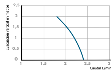
SANICONDENS® Mini
